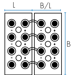
20 OPzS 2500 - 26 OPzS 3250
